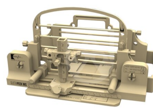
Urządzenie do biopsji piersi wykonane z materiału SUSTAPEEK MG
